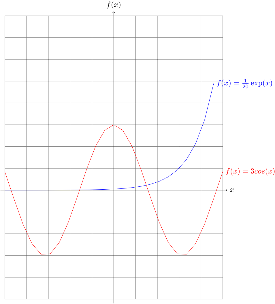
FIGURE 2 – Des fonctions
