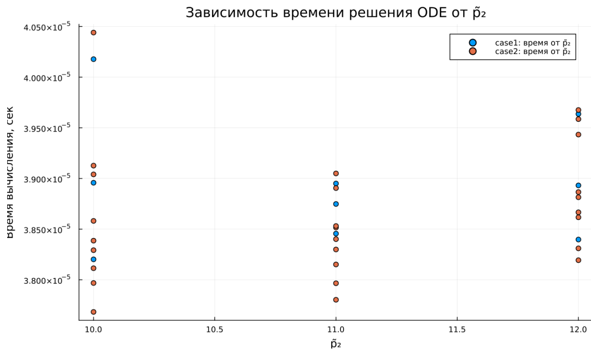
Рисунок 5.24: Зависимость времени решения ODE от \tilde{p}_2
