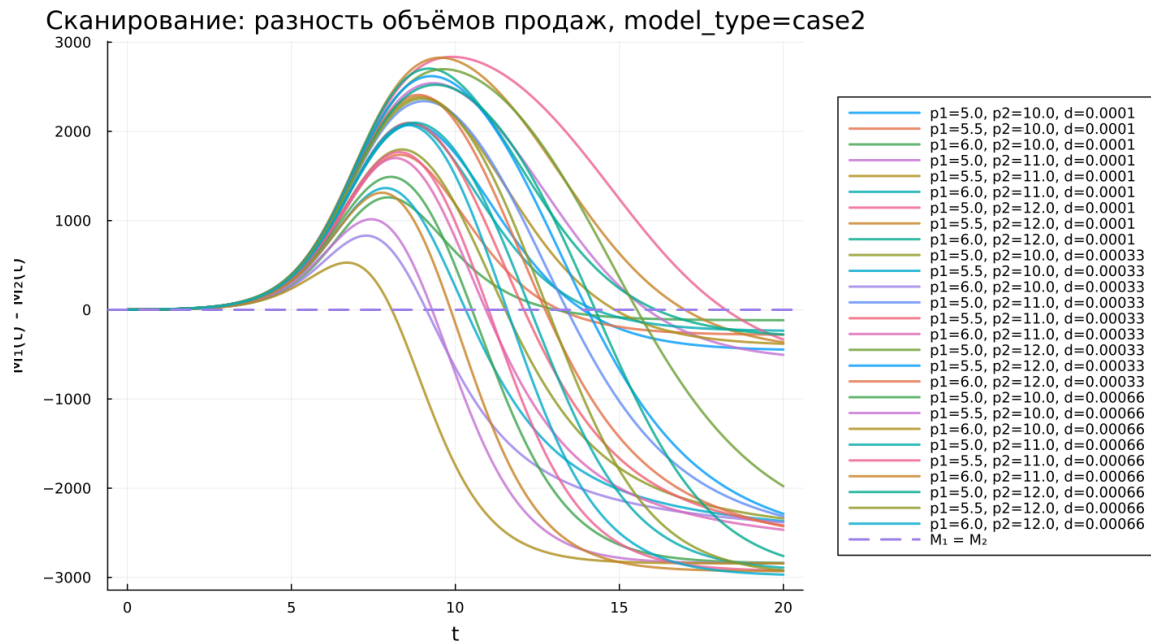
Рисунок 5.10: Сканирование: разность объёмов продаж, вторая модель
