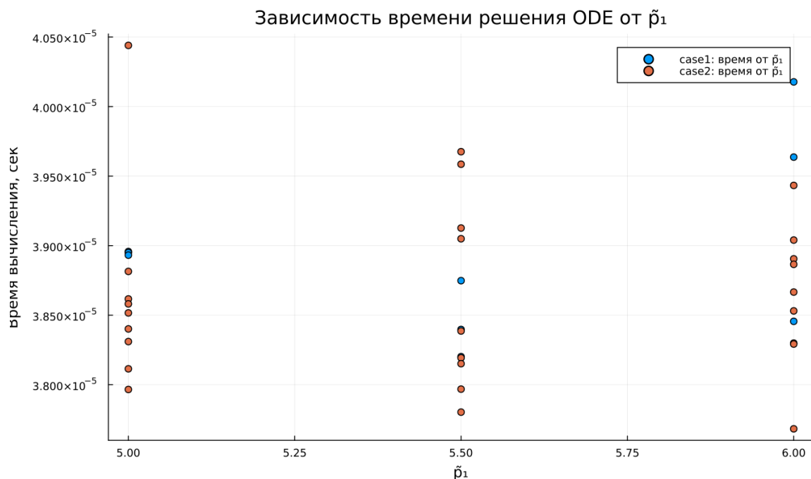
Рисунок 5.23: Зависимость времени решения ODE от p_1
