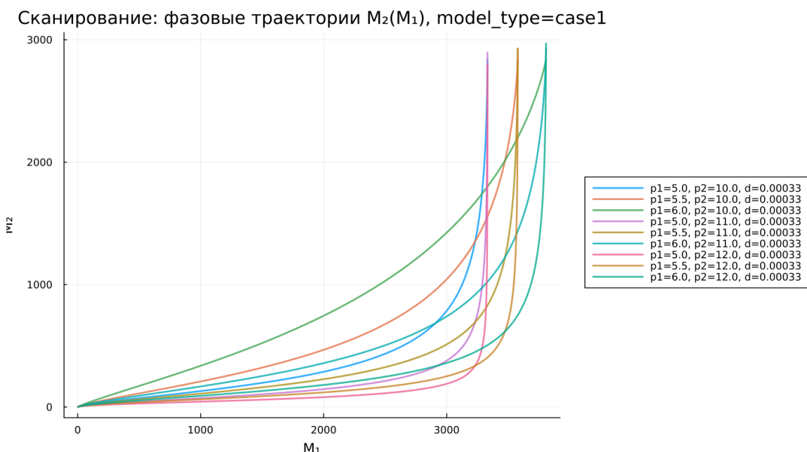
Рисунок 5.15: Сканирование: фазовые траектории M_2(M_1) , первая модель
