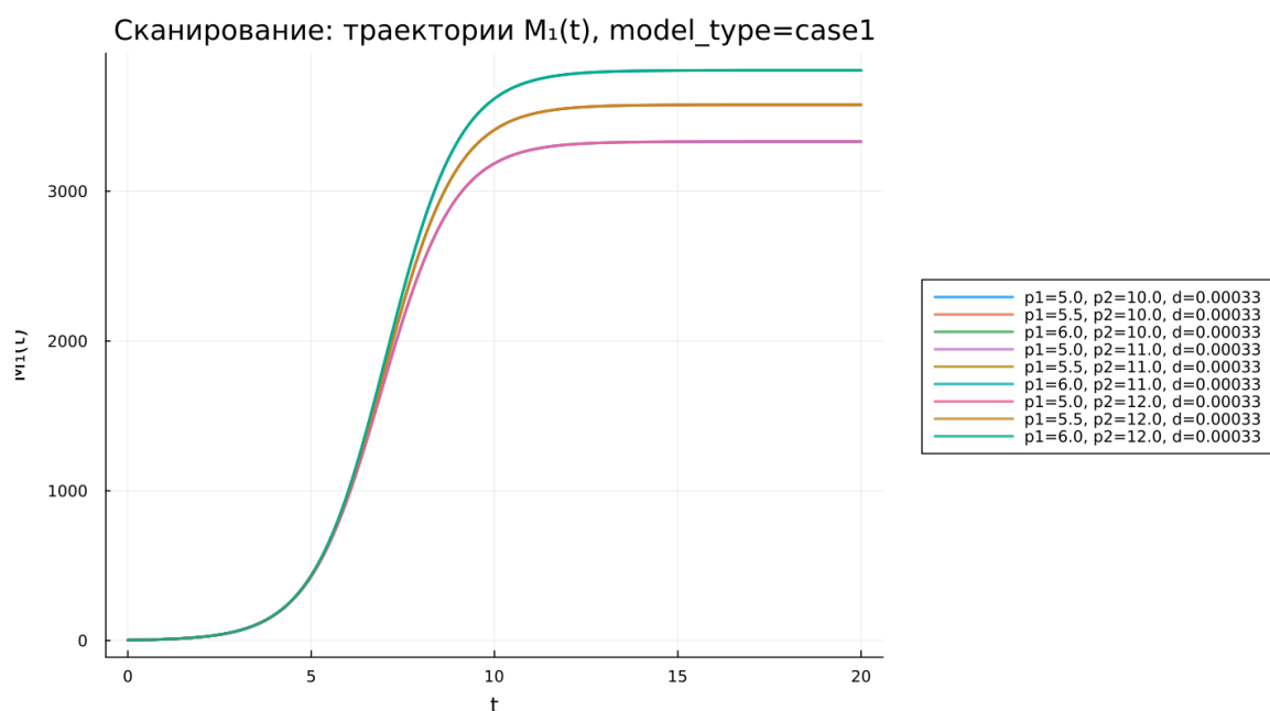
Рисунок 5.11: Сканирование: траектории M_1(t) , первая модель
