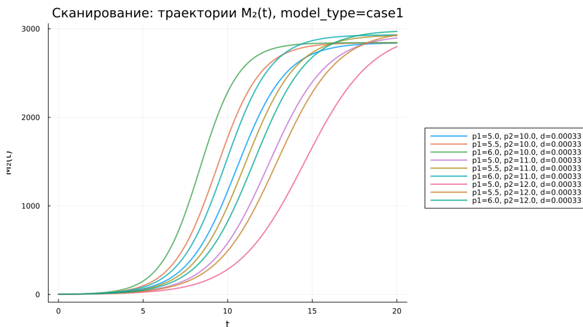
Рисунок 5.13: Сканирование: траектории M_2(t) , первая модель
