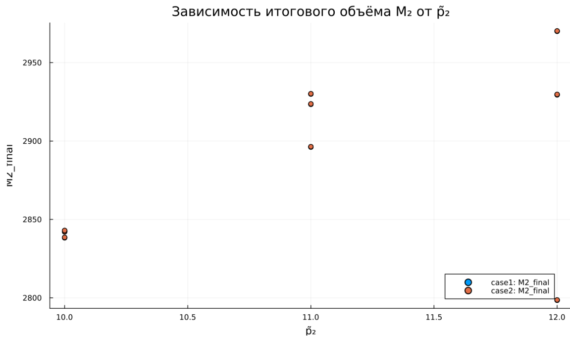
Рисунок 5.21: Зависимость итогового объёма M_2 от p_2
