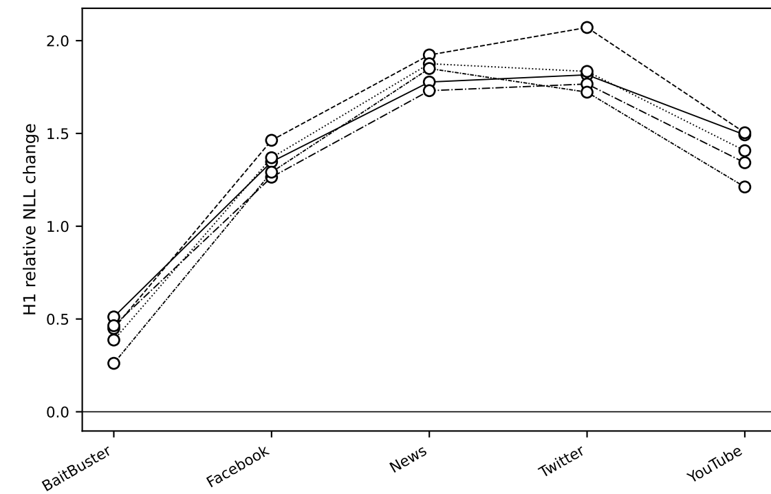
XLM-R
