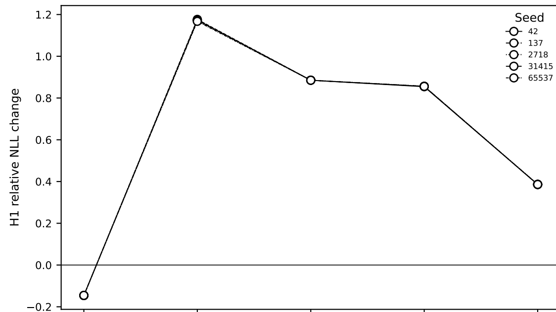
BanglaBERT
