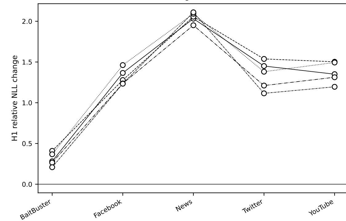
BanglaBERT
