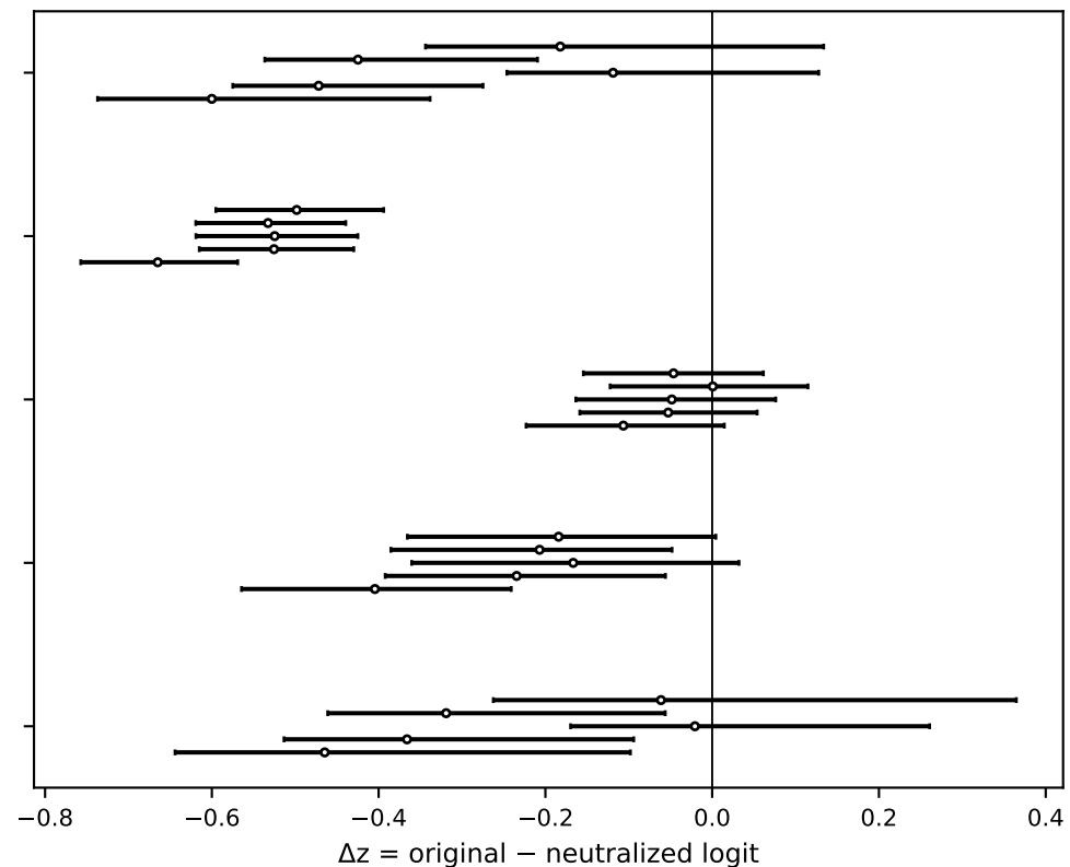
BanglaBERT
