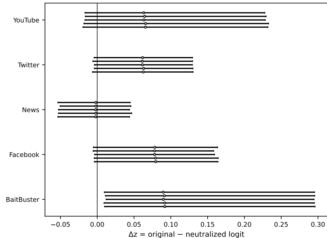
EBM
