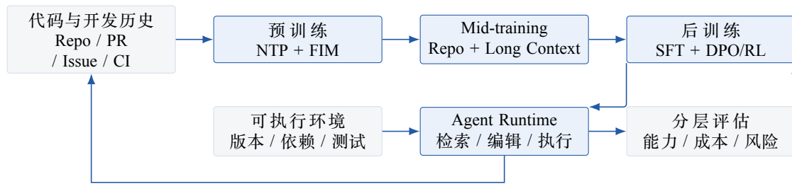
图 1: Code Agent 的四线闭环。训练数据必须保留到可执行环境与评估结果的血缘，运行轨迹再回流为下一轮 SFT、偏好或 verifier 数据。
