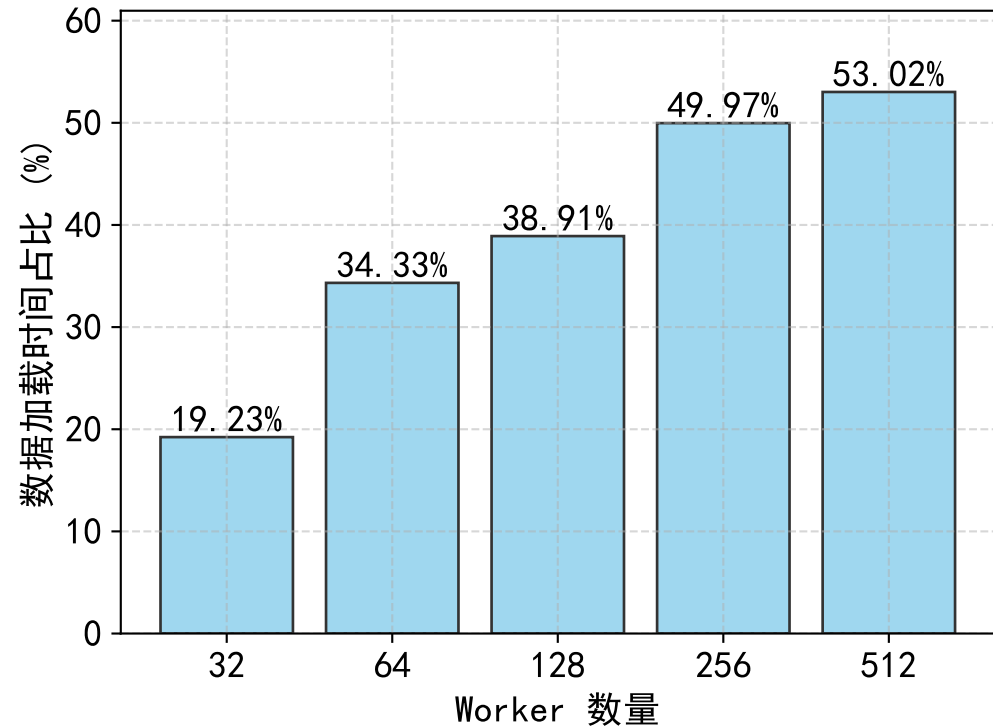
单机单 GPU 数据加载时间占比
