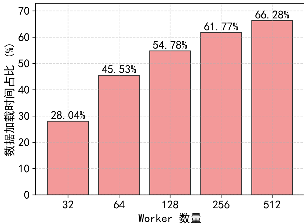
单机双 GPU 数据加载时间占比
