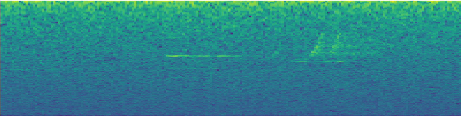
(b) Log+median
