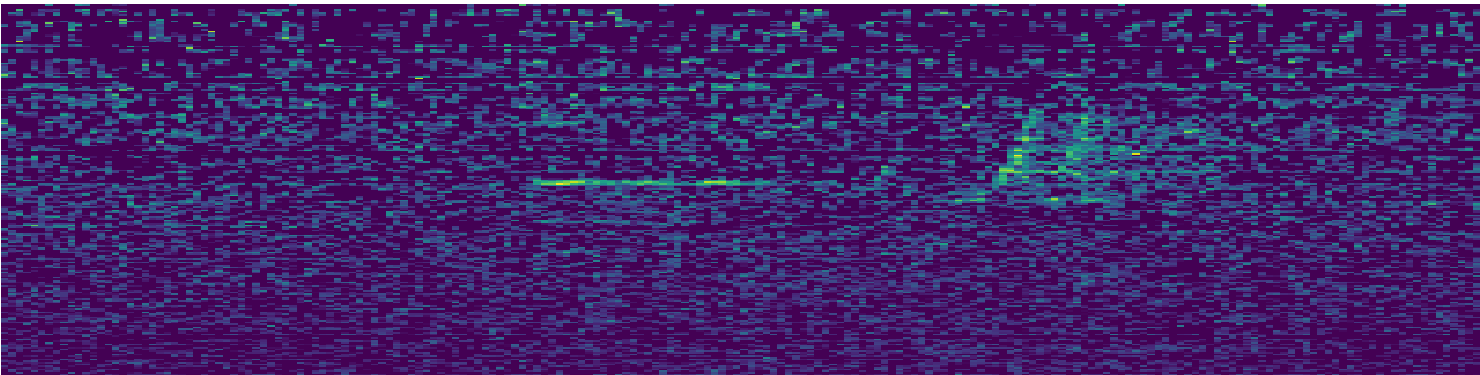
(d) Log+normalize+median
