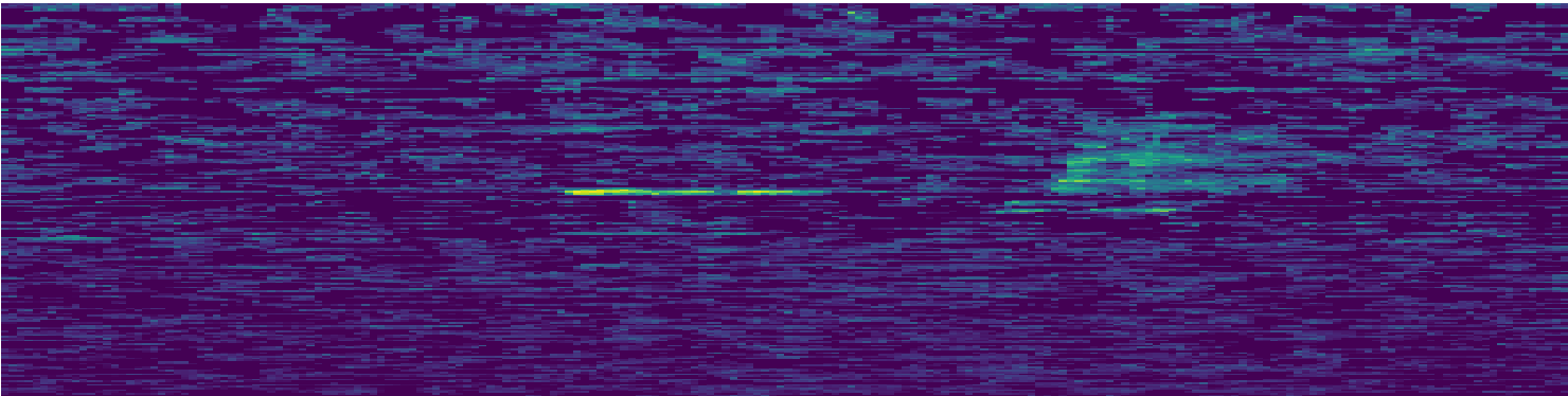
(e) PCEN
