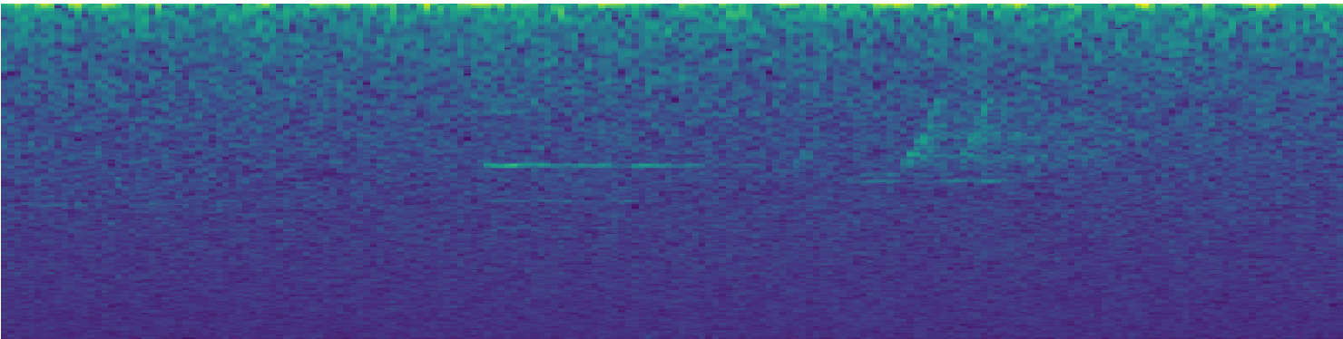
(f) Box-Cox
