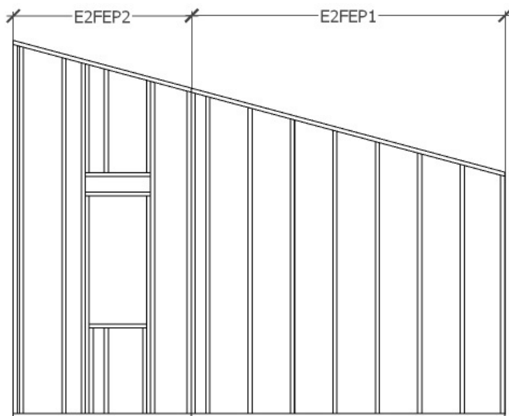
VISTA GENERAL — FACHADA ESTE ETAPA 2
