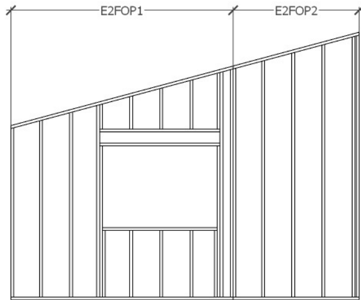
VISTA GENERAL — FACHADA OESTE ETAPA 2
