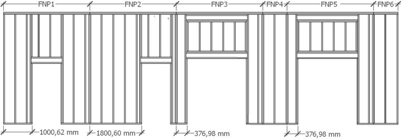
VISTA GENERAL — FACHADA NORTE COMPLETA
