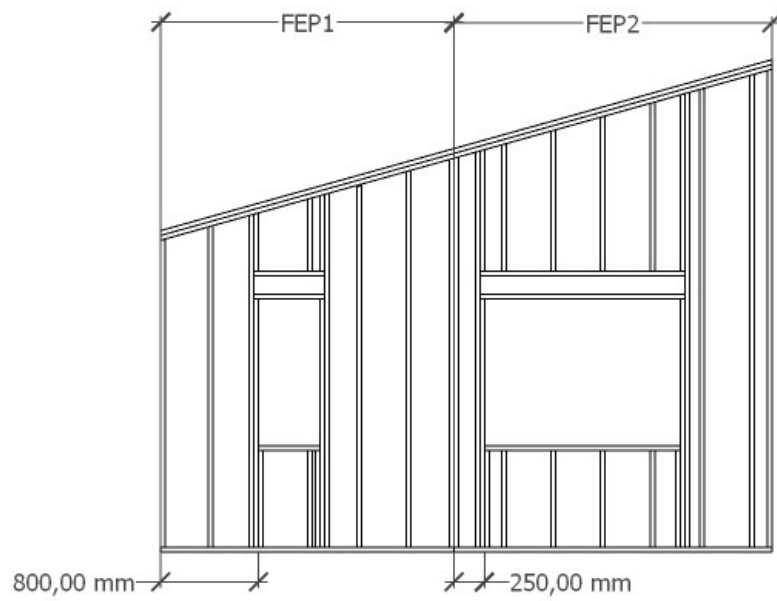
VISTA GENERAL — FACHADA ESTE COMPLETA
