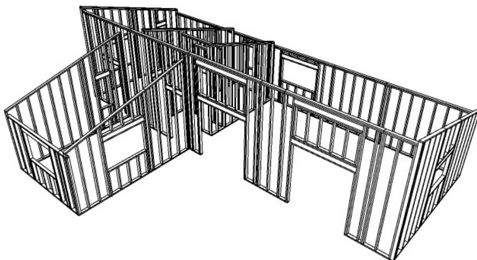
VISTA EN ÁNGULO — ESTRUCTURA COMPLETA
