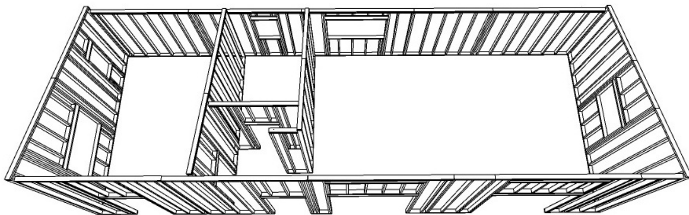
VISTA DESDE ARRIBA — ESTRUCTURA COMPLETA
