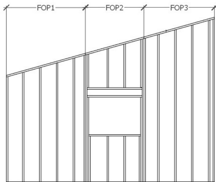
VISTA GENERAL — FACHADA OESTE COMPLETA
