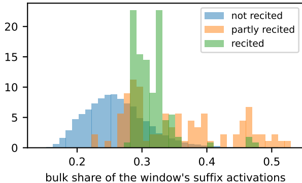
OLMo-3 7B, layer 23 input, AUC 0.84
