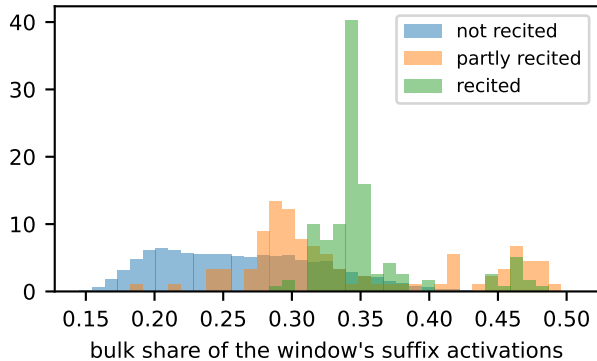
OLMo-2 7B, layer 23 input, AUC 0.89
