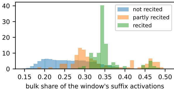
OLMo-2 7B, layer 23 input, AUC 0.89
