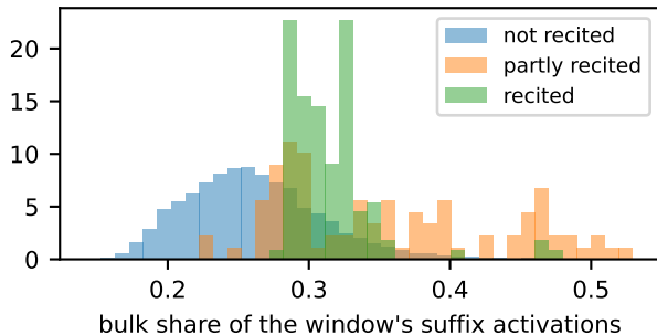
OLMo-3 7B, layer 23 input, AUC 0.84
