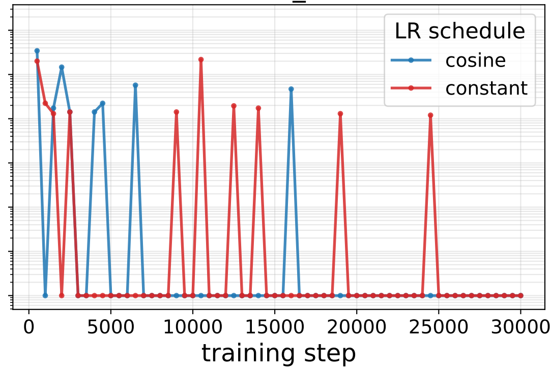
sokoban_basic
