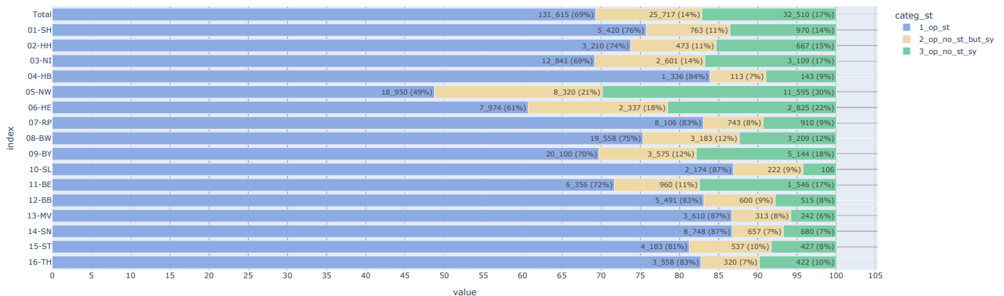
ST Kategorien nach OP mit BET bei C50, n=189_842
