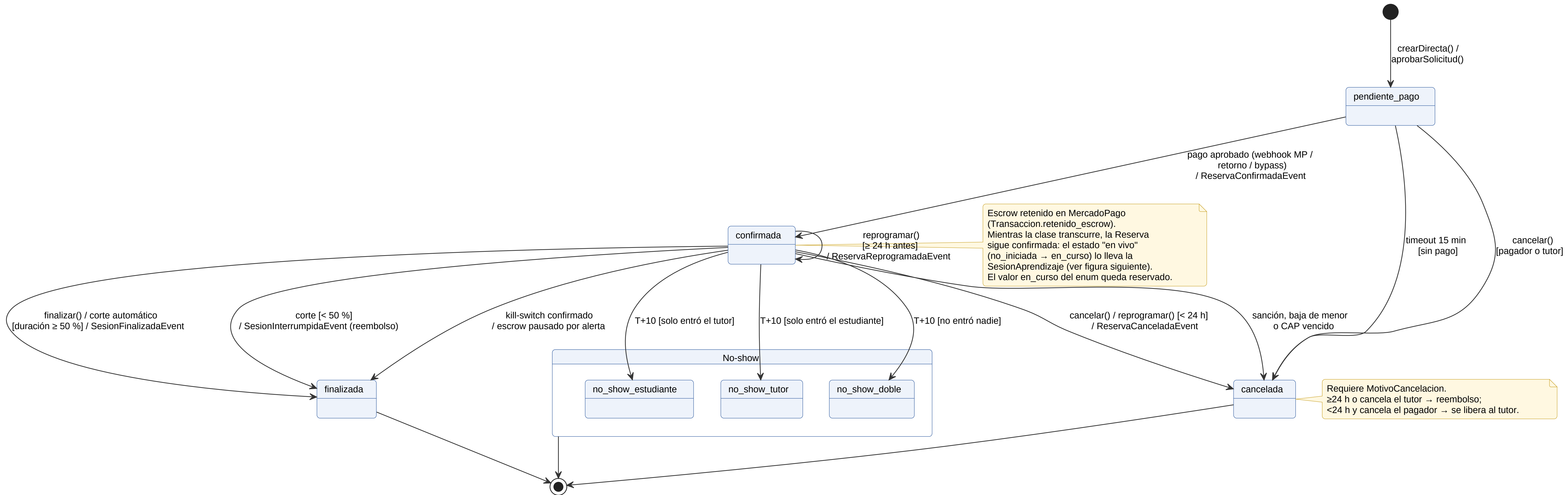
Diagrama de máquina de estados — Reserva (EstadoReserva)
