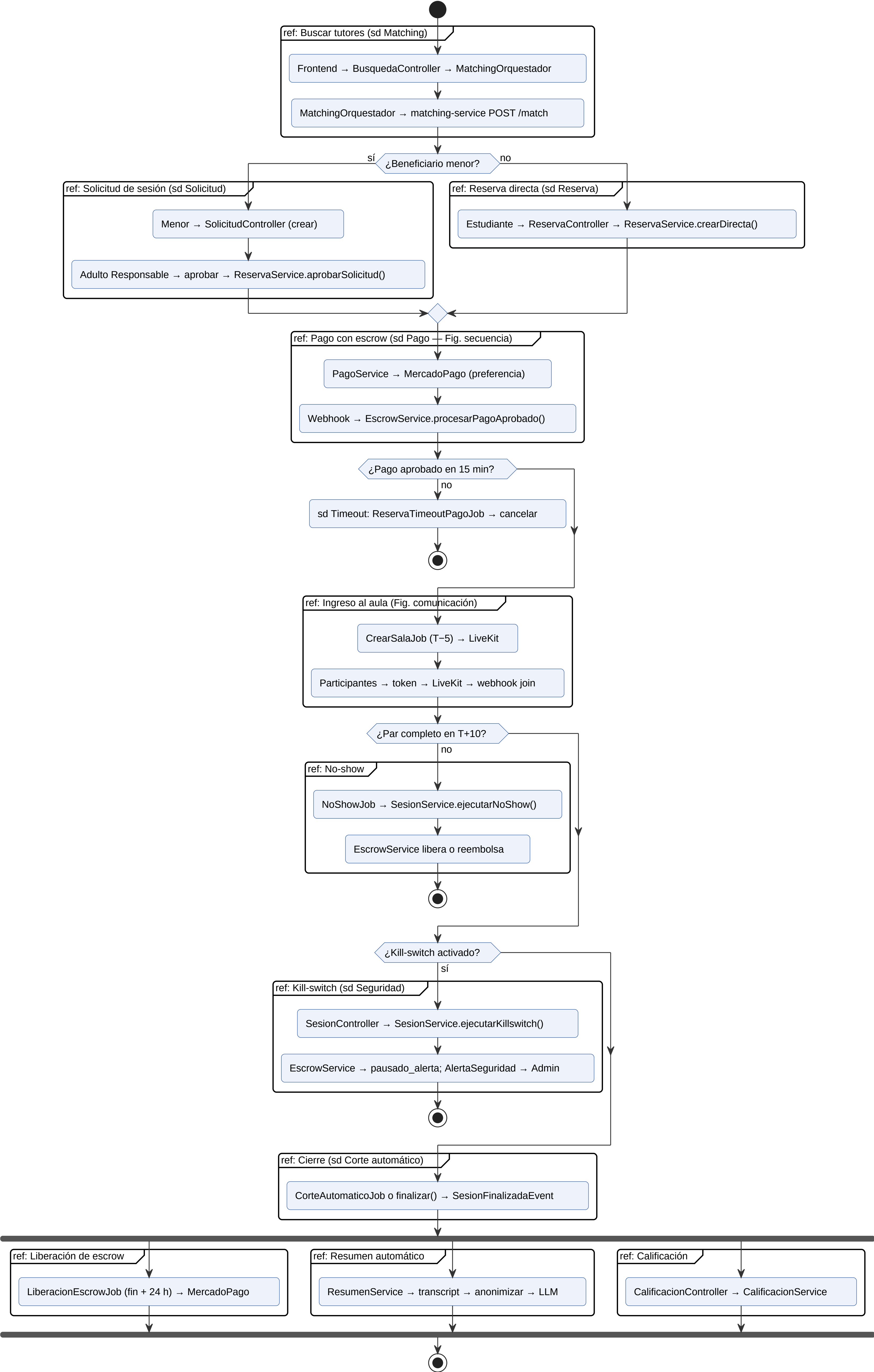
Diagrama de visión general de interacciones — De la búsqueda al cierre de la clase
