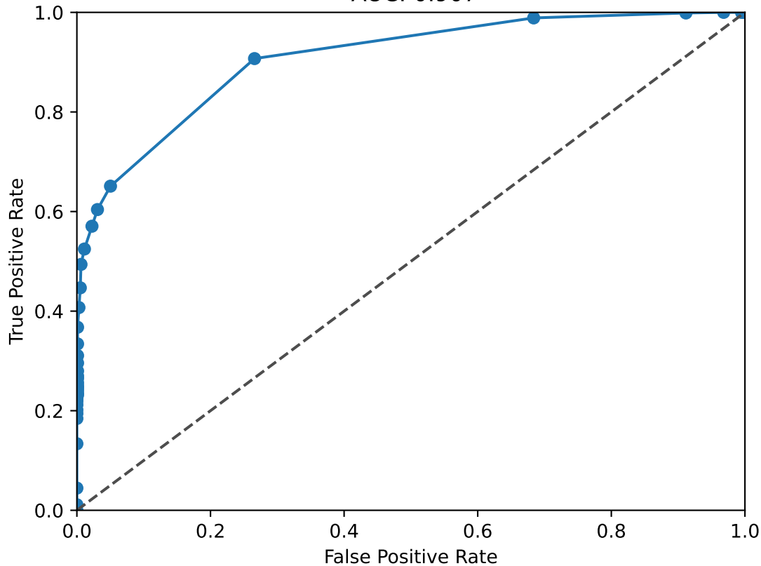
BACH2 ROC Curve AUC: 0.907
