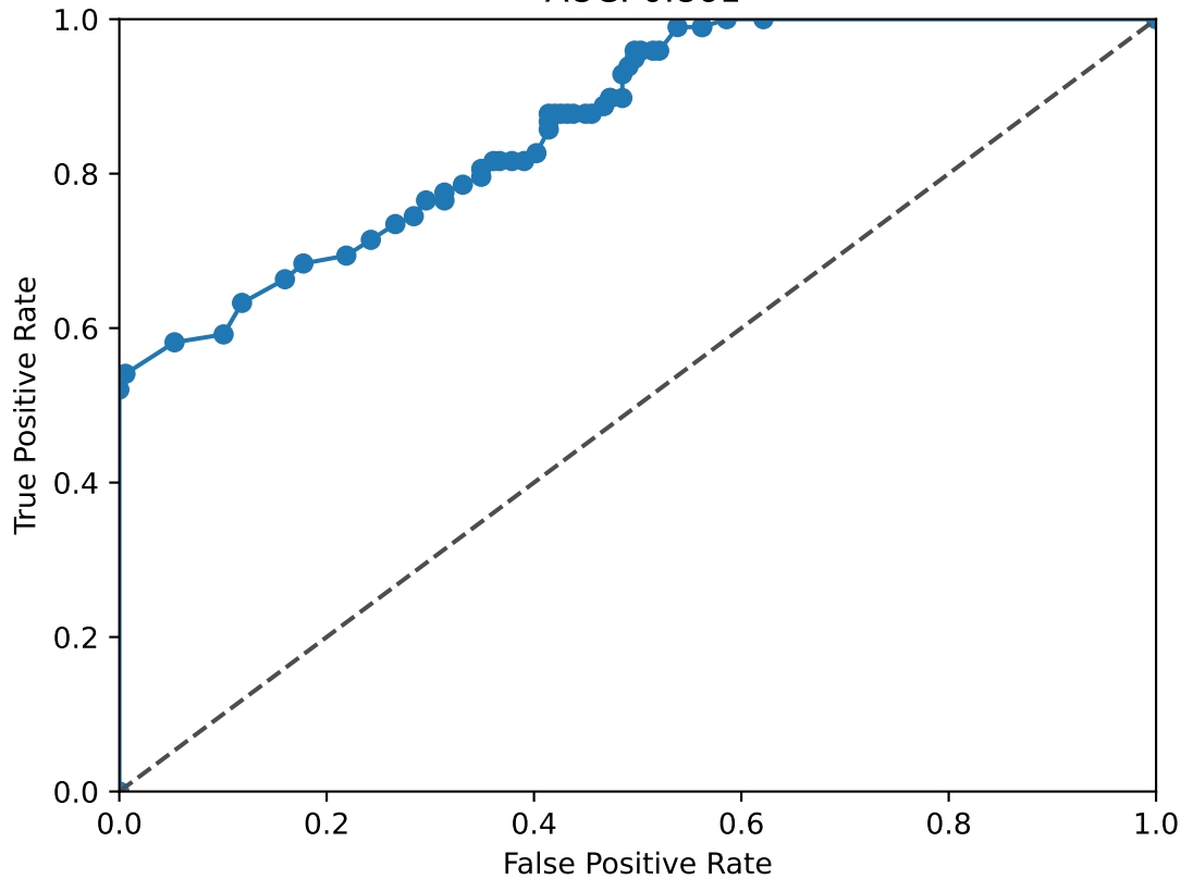
ZBTB20 ROC Curve AUC: 0.861
