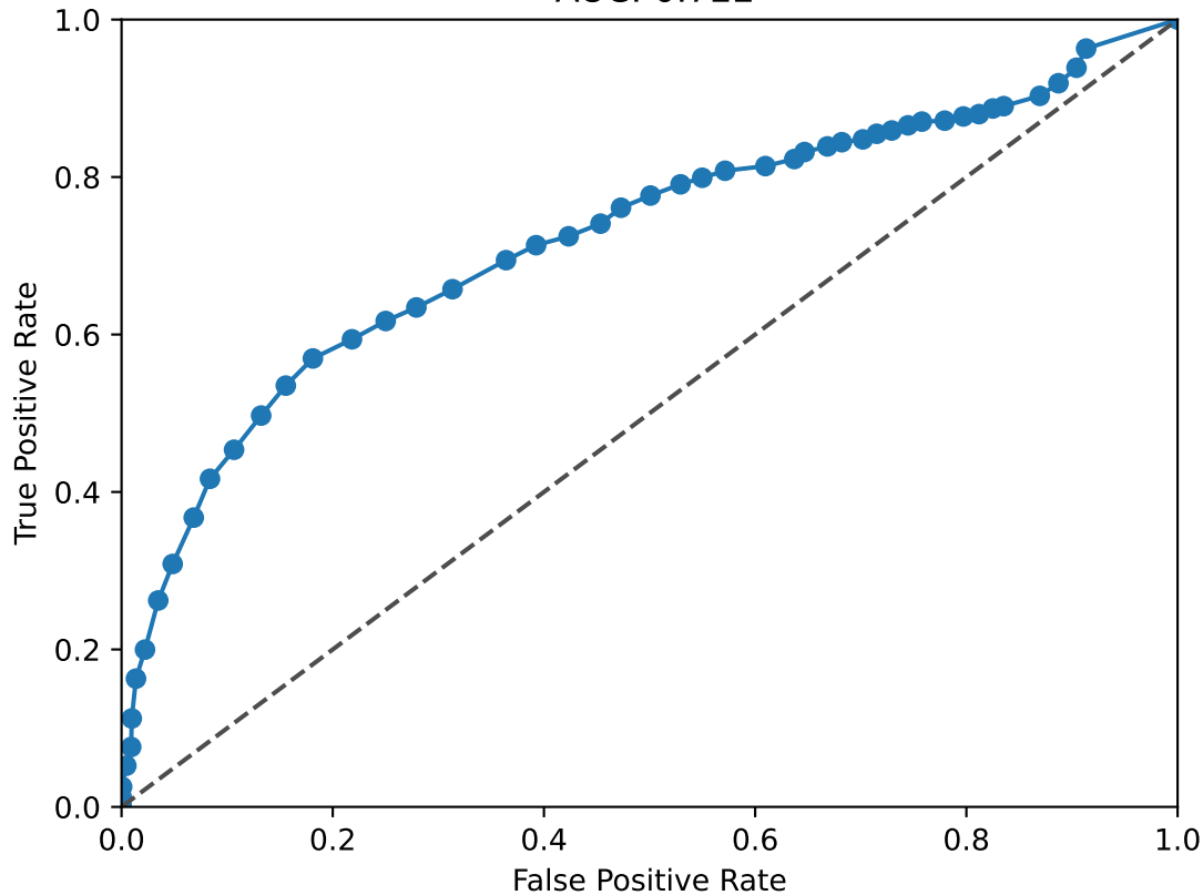
ZBTB20 ROC Curve AUC: 0.722
