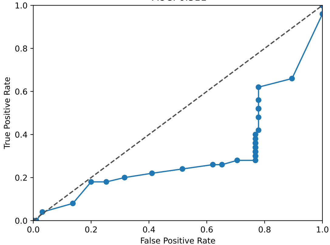
AUC: 0.311
