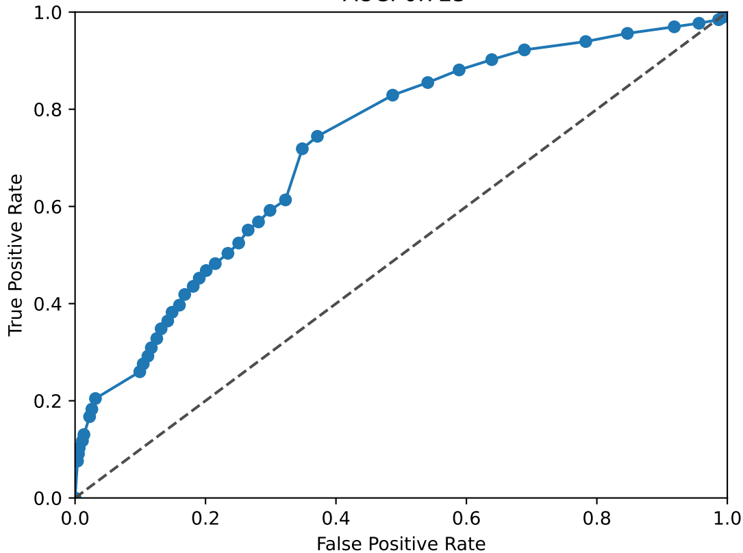
BACH2 ROC Curve AUC: 0.723
