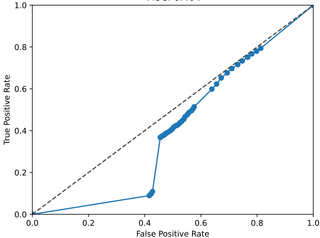
EHF ROC Curve AUC: 0.404
