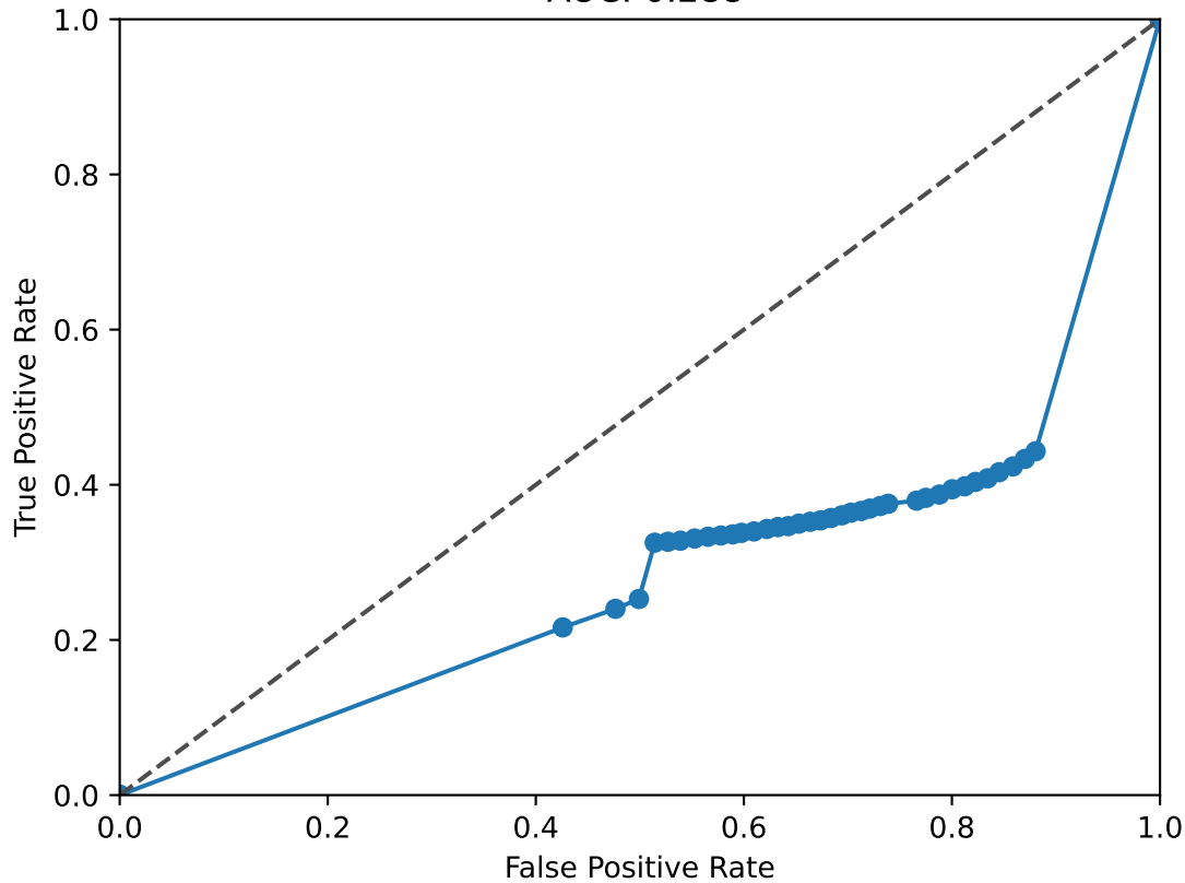
EHF ROC Curve AUC: 0.288
