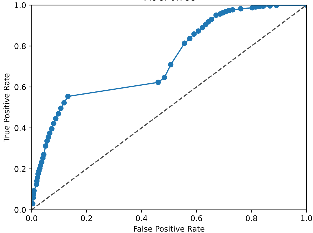
ZBTB20 ROC Curve AUC: 0.733
