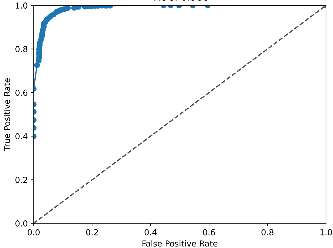
LMX1B ROC Curve AUC: 0.988
