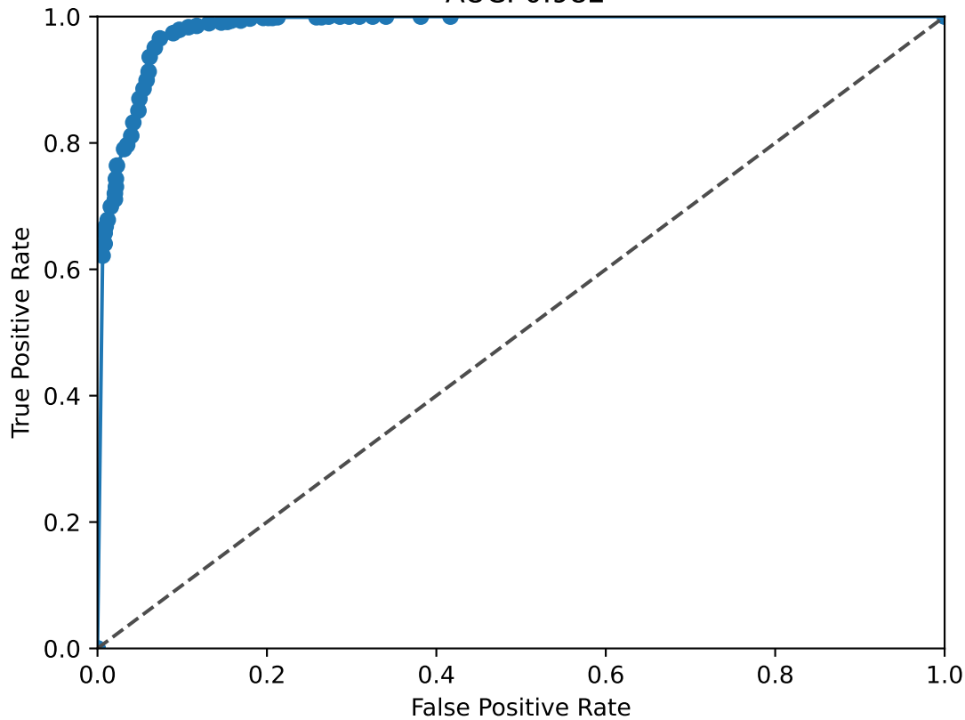
MEIS2 ROC Curve AUC: 0.982
