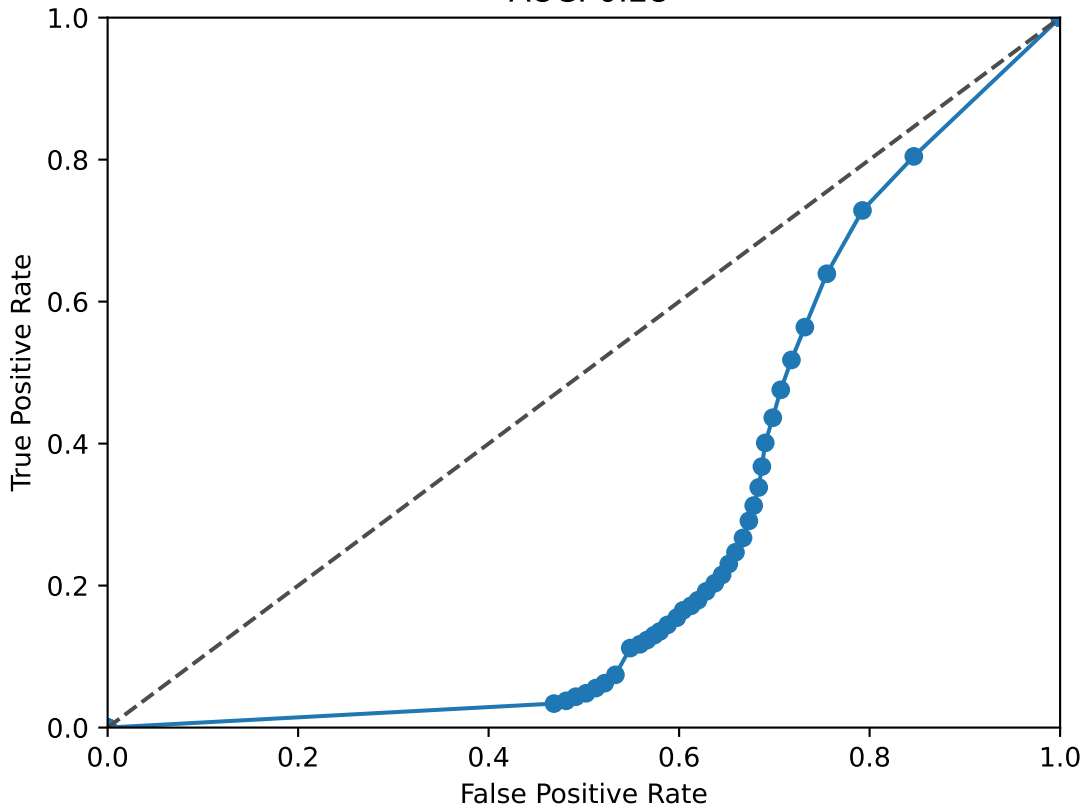
EHF ROC Curve AUC: 0.28
