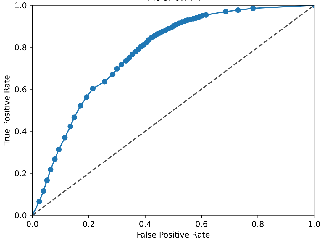
MEIS2 ROC Curve AUC: 0.774
