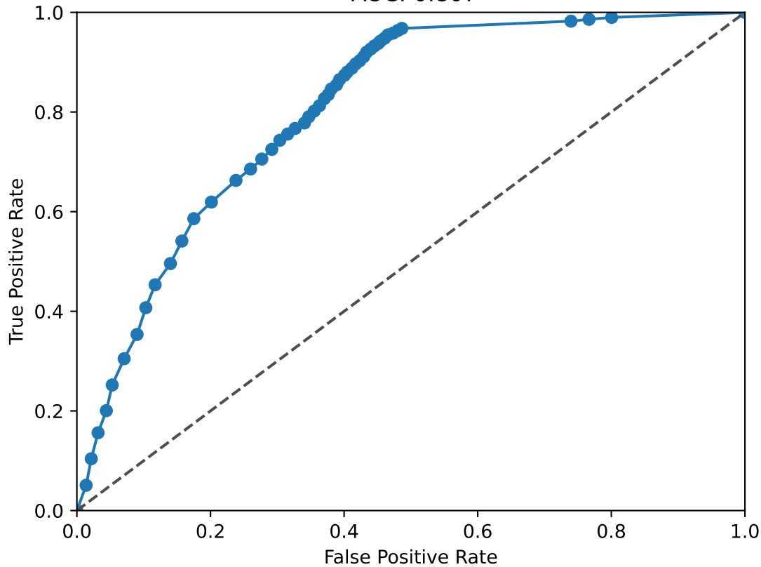
MEIS2 ROC Curve AUC: 0.807
