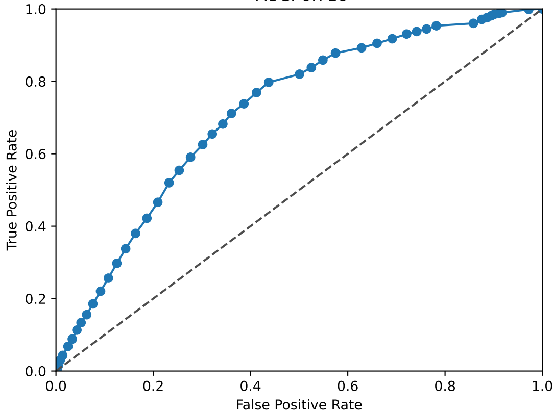
ZBTB20 ROC Curve AUC: 0.716
