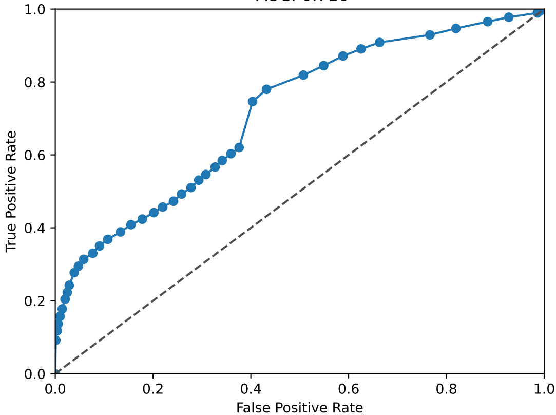
BACH2 ROC Curve AUC: 0.716
