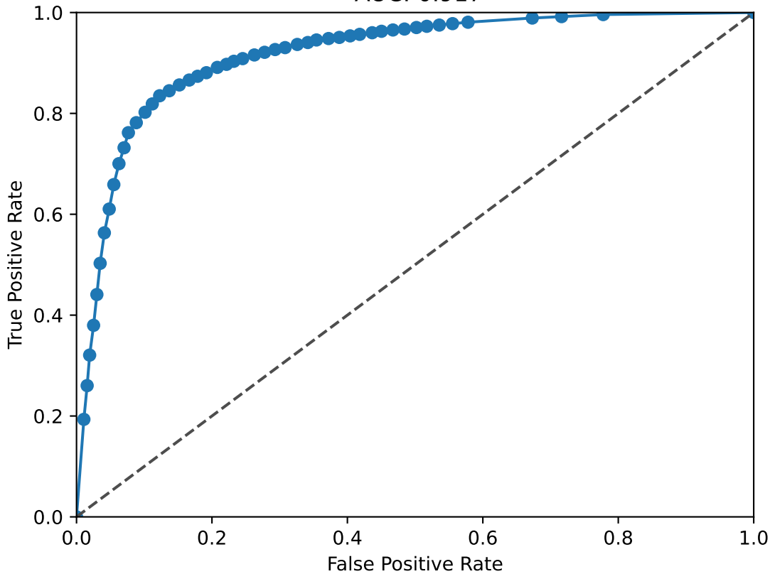
MEIS2 ROC Curve AUC: 0.917
