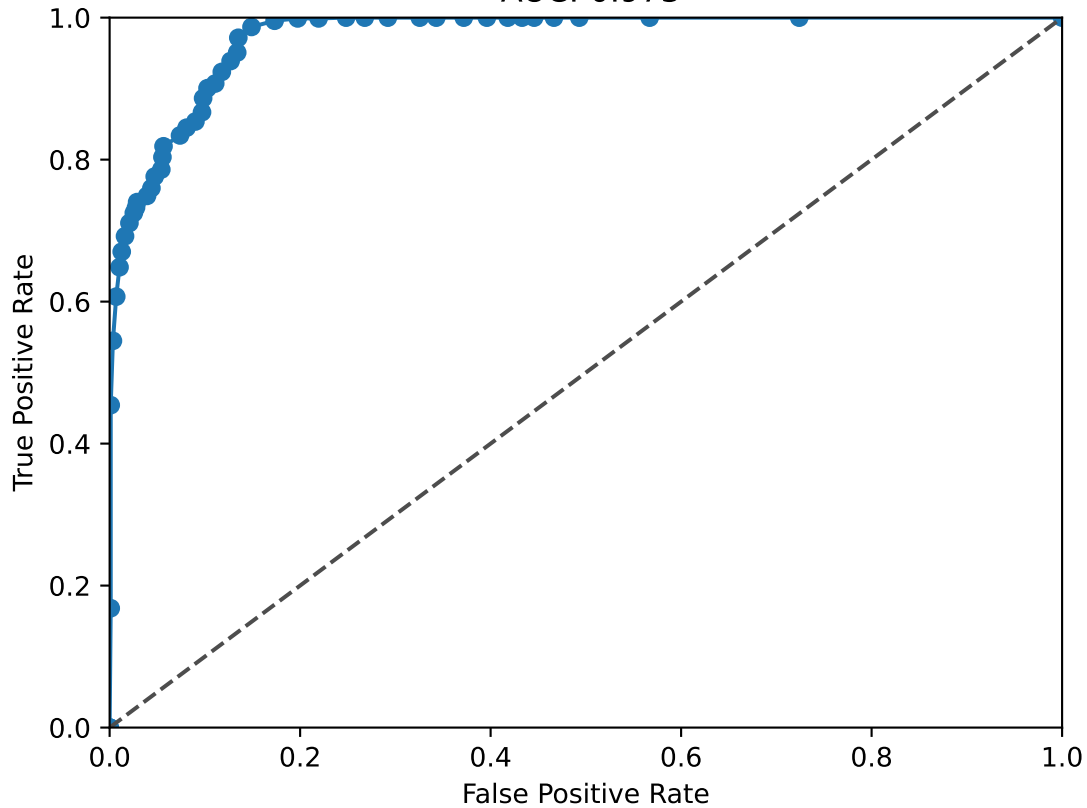
MEIS2 ROC Curve AUC: 0.973
