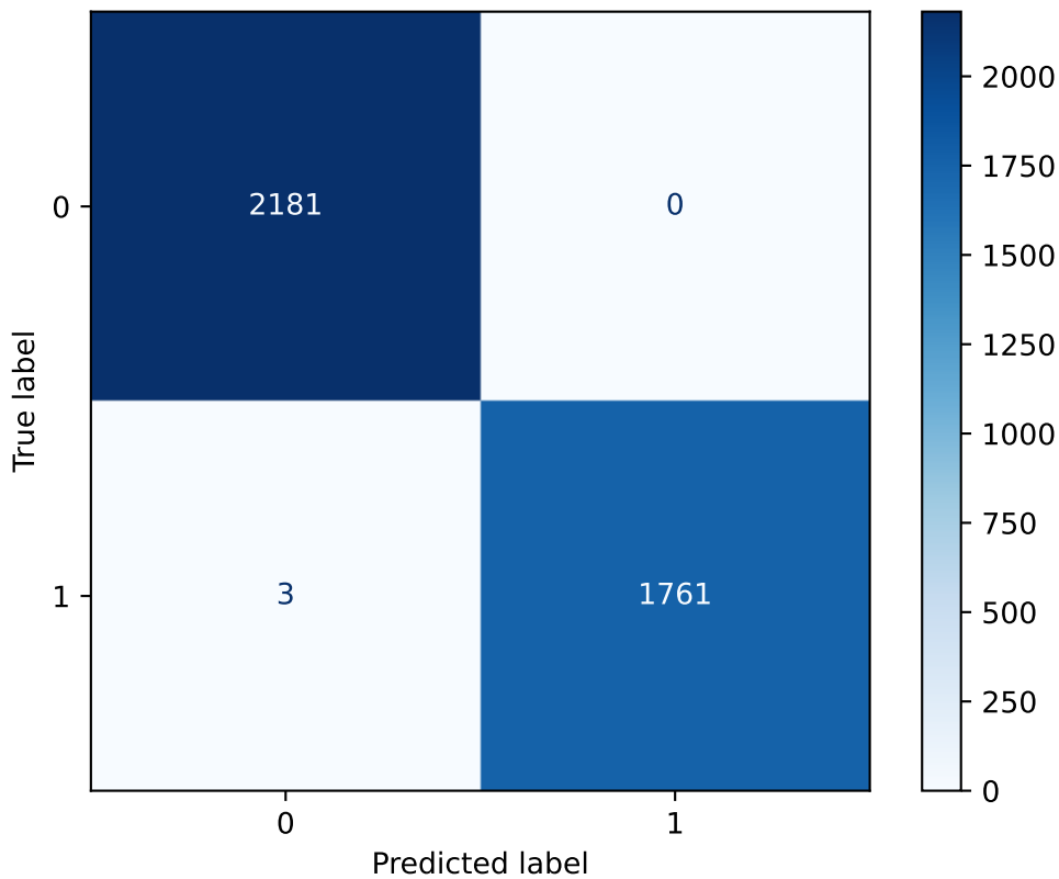
CREB1
