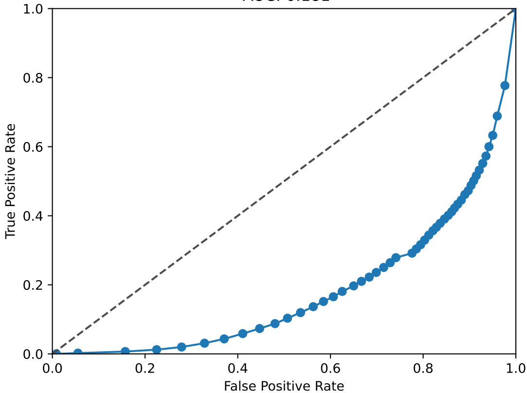
NFIB ROC Curve AUC: 0.181
