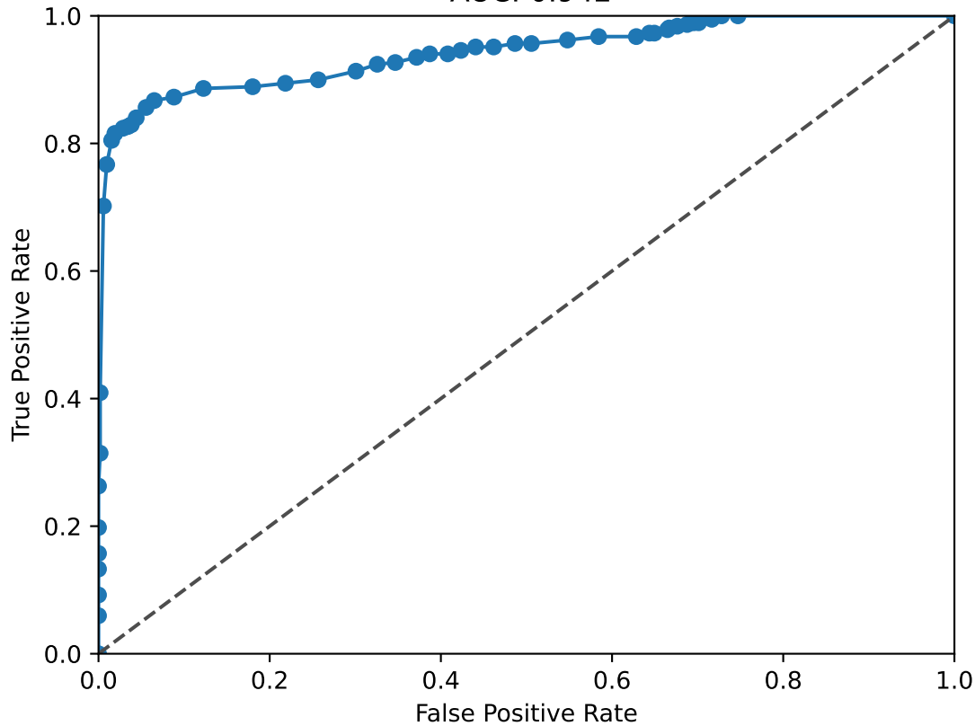
ZBTB20 ROC Curve AUC: 0.942
