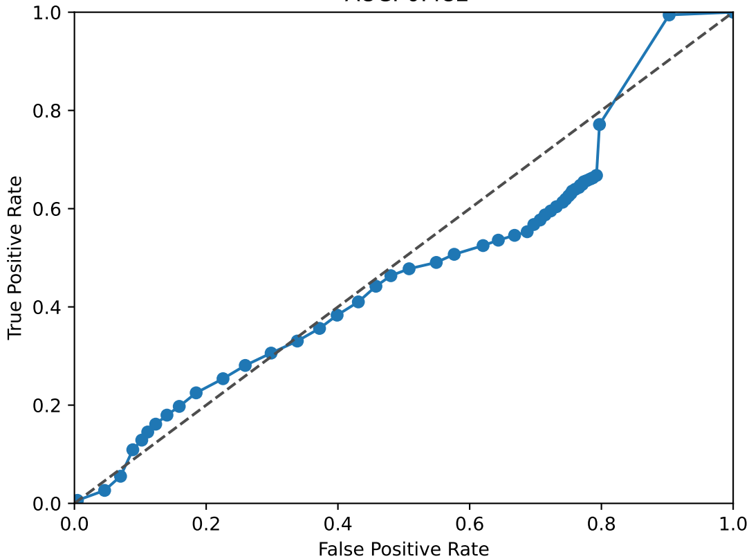
NFIA ROC Curve AUC: 0.482
