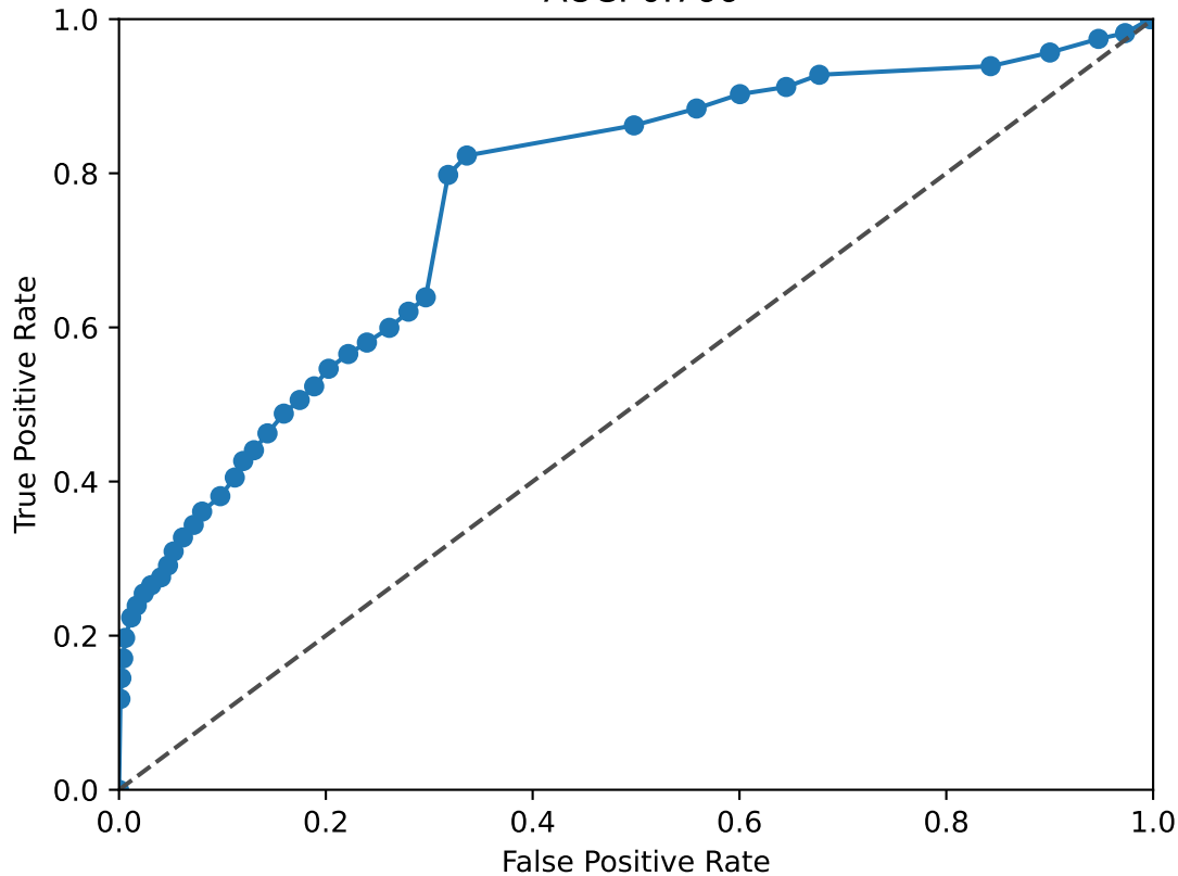
BACH2 ROC Curve AUC: 0.766
