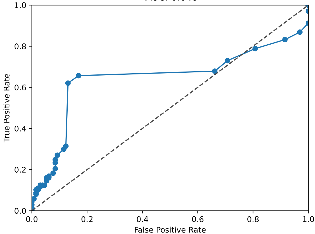
BACH2 ROC Curve AUC: 0.648
