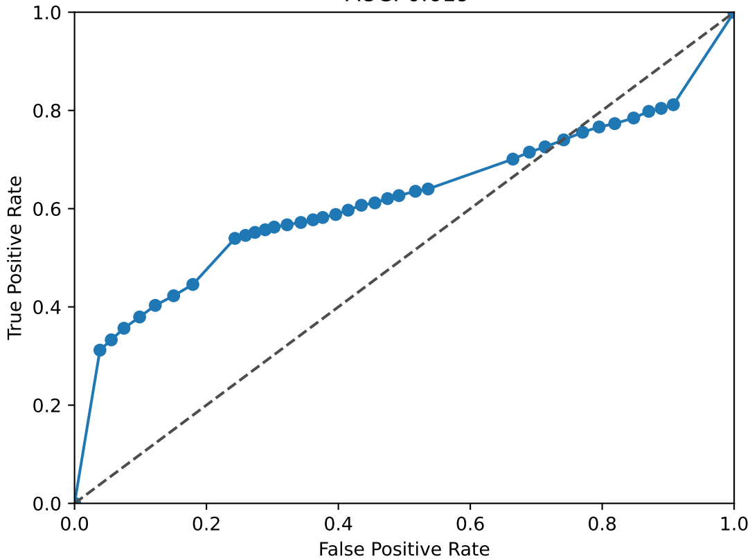
EHF ROC Curve AUC: 0.619
