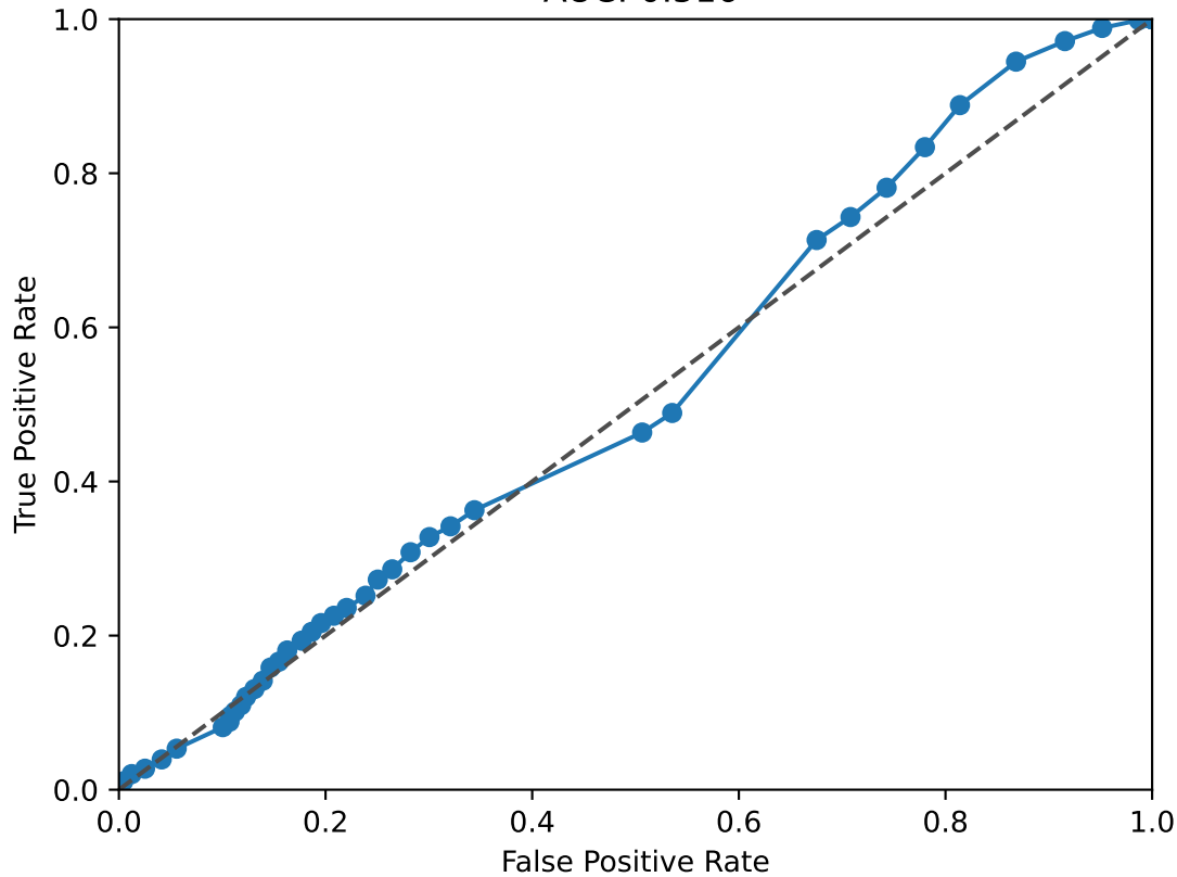
BACH2 ROC Curve AUC: 0.516
