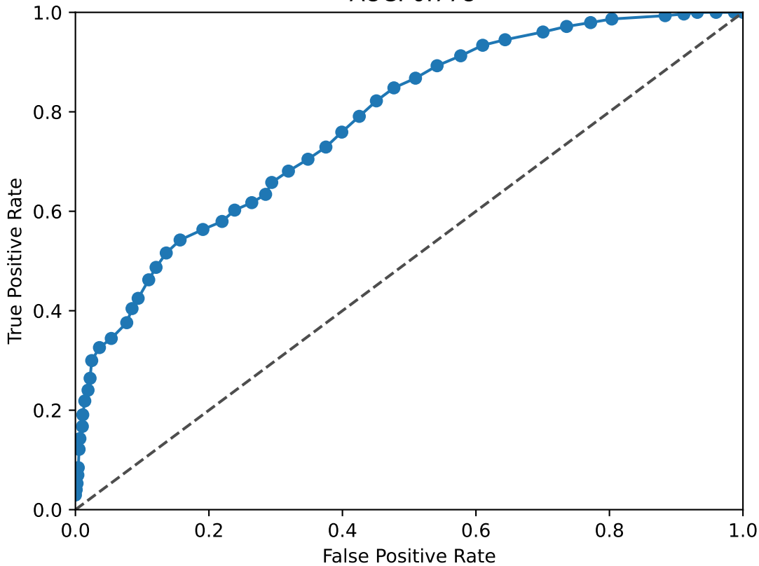
NFIA ROC Curve AUC: 0.778
