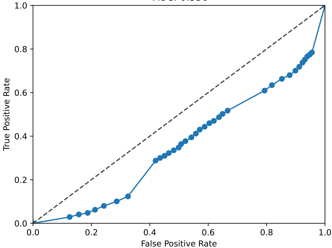
EHF ROC Curve AUC: 0.356
