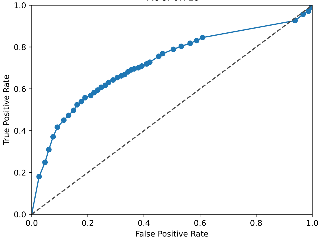
BACH2 ROC Curve AUC: 0.719
