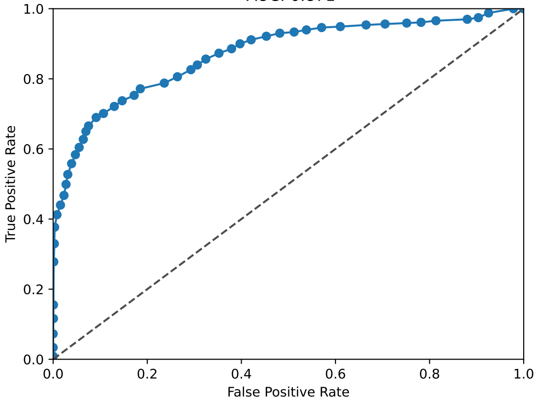
ZBTB20 ROC Curve AUC: 0.871
