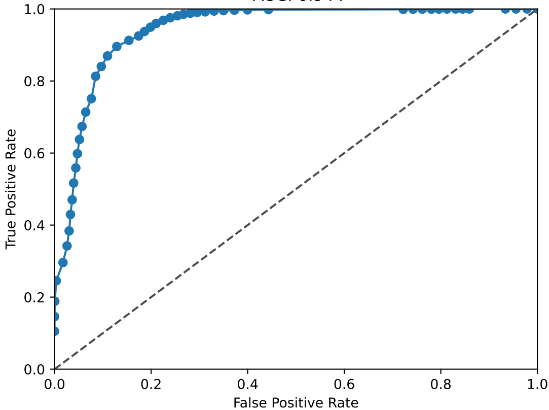
LMX1B ROC Curve AUC: 0.944
