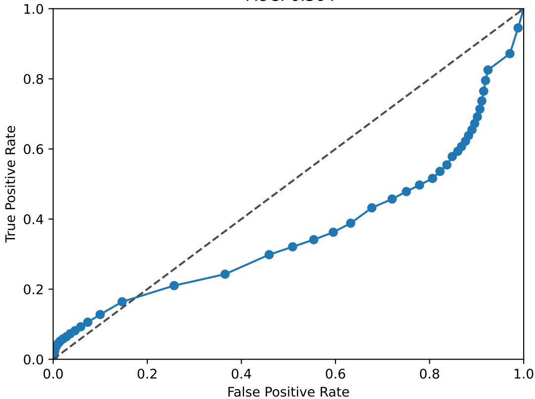
NFIA ROC Curve AUC: 0.364
