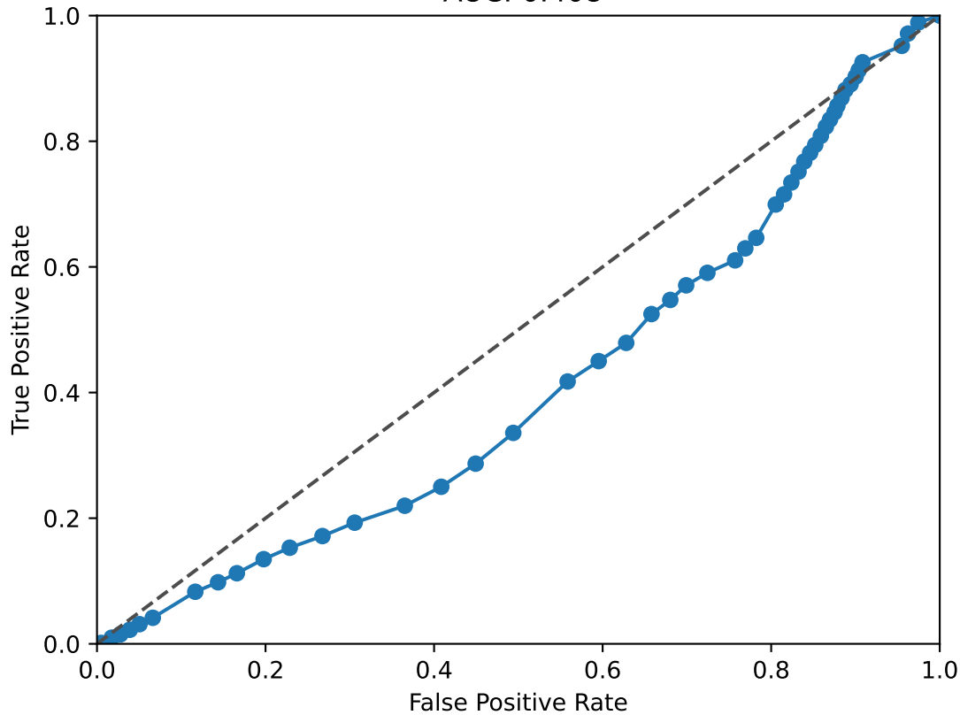
MEIS2 ROC Curve AUC: 0.408
