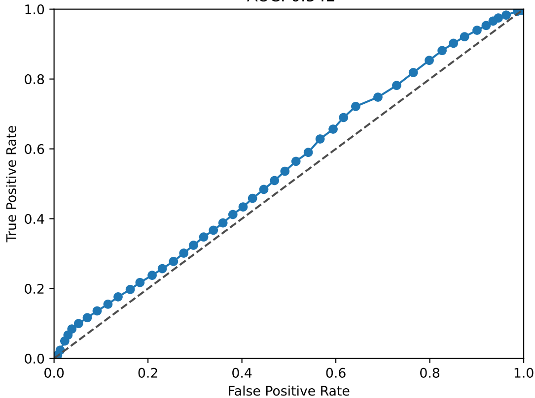
ZBTB20 ROC Curve AUC: 0.542
