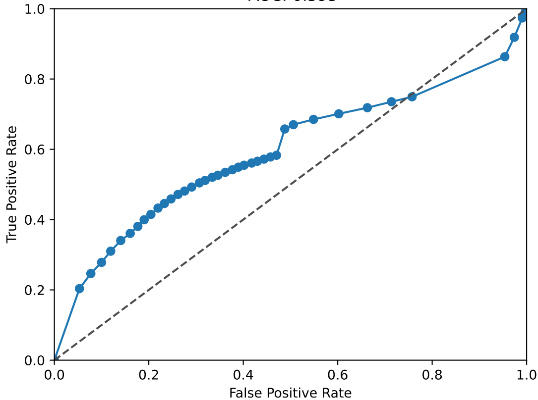
BACH2 ROC Curve AUC: 0.593
