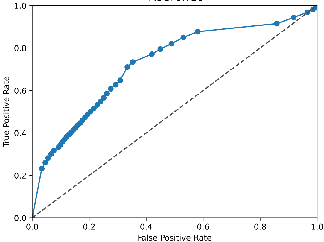
BACH2 ROC Curve AUC: 0.726
